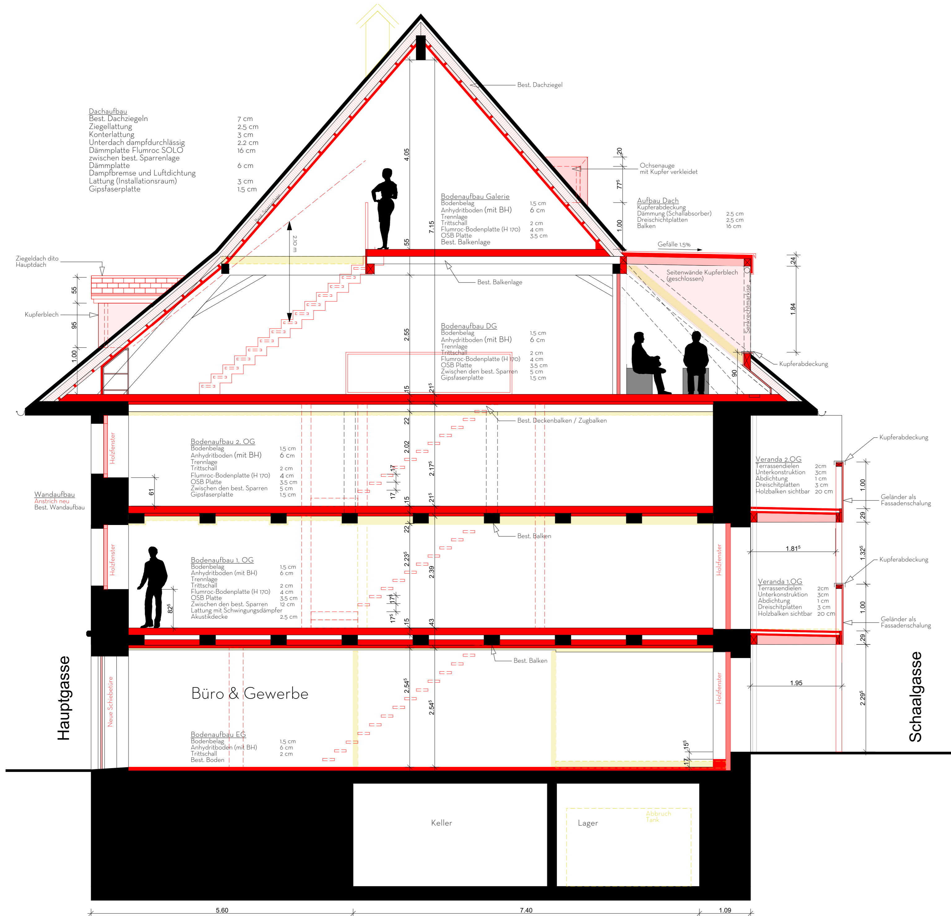
Schnitt - Mst.: 1:50
