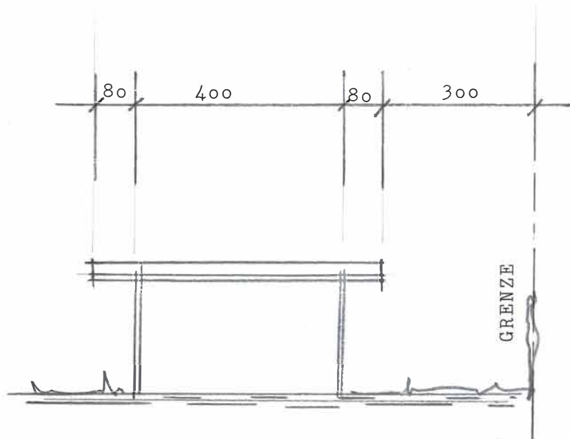
NORDSEITE MST. 1:100
