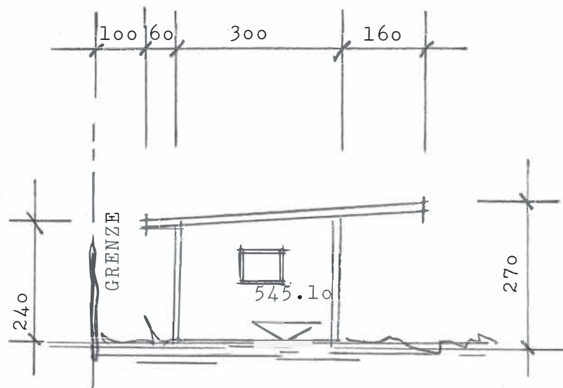
WESTSEITE MST. 1:100
