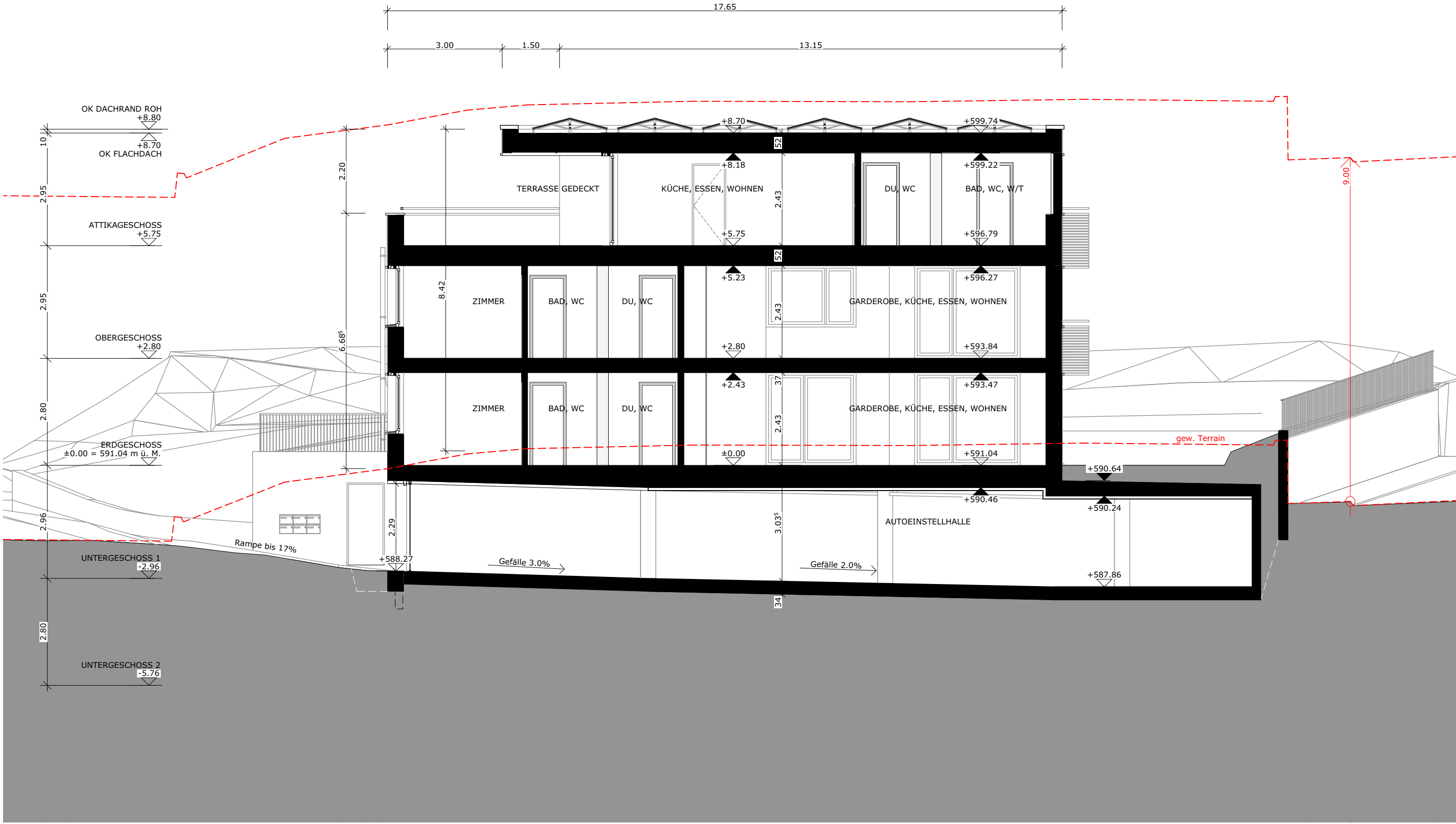
SCHNITT C
