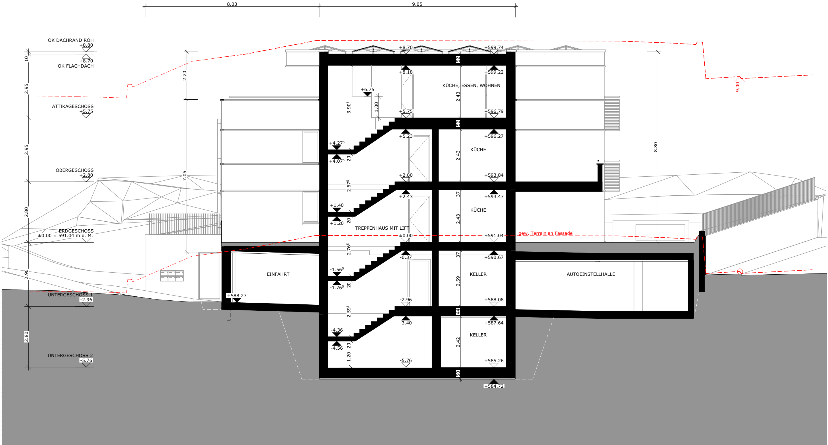
SCHNITT B
