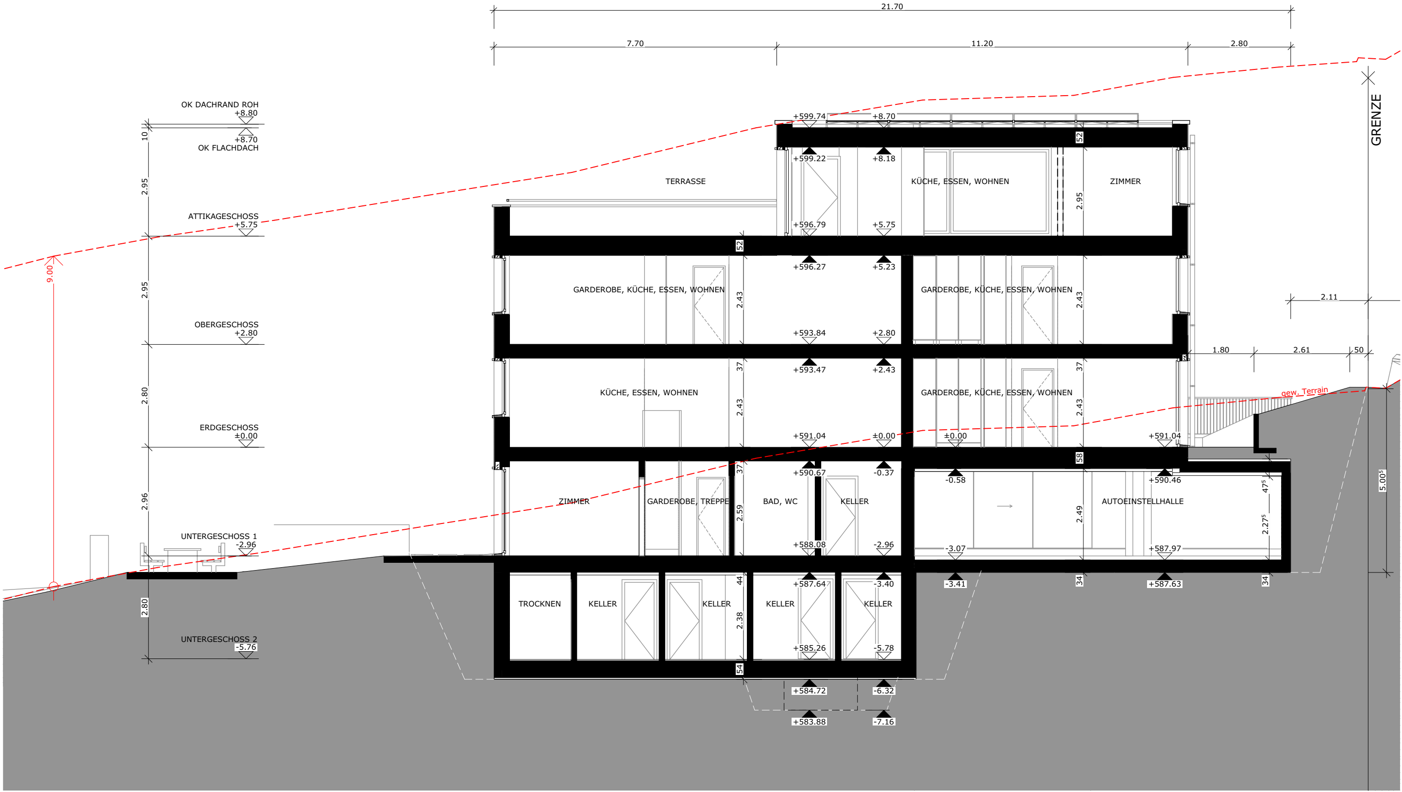
SCHNITT D
